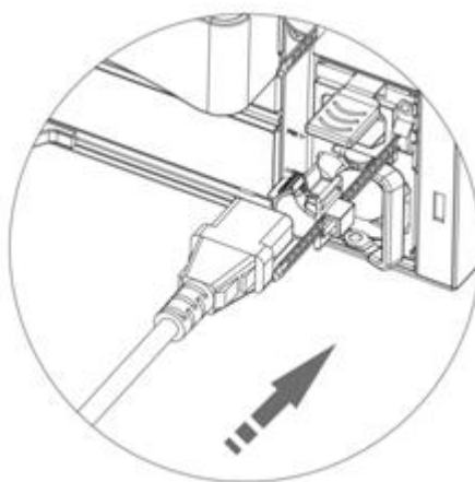
图4-31 安装电源线示意图（一）
