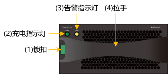
图3-24 DSU2624B 风扇模块+电池模块正视图
