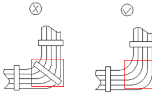
图4-25 线缆捆扎示意图（三）
