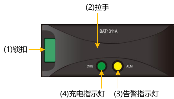
图3-7 SPU 电池模块正视图
