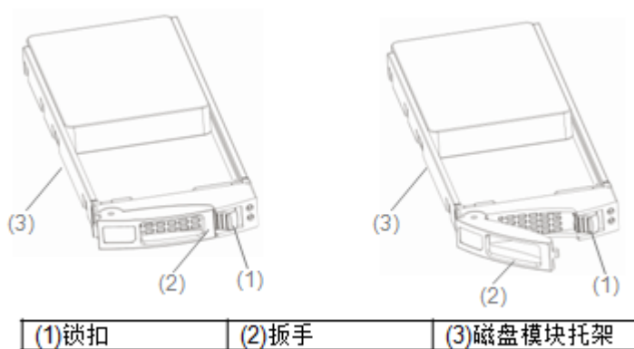
图6-34 NVMe 磁盘模块示意图
