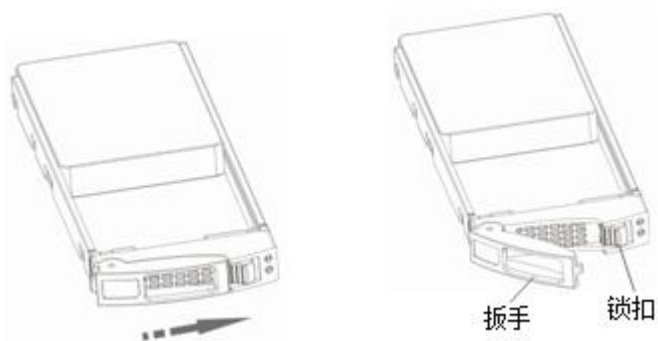
图6-36 安装 NVMe 磁盘模块示意图（一）
