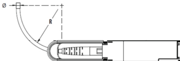
图4-38 AOC 光缆弯曲半径示意图
