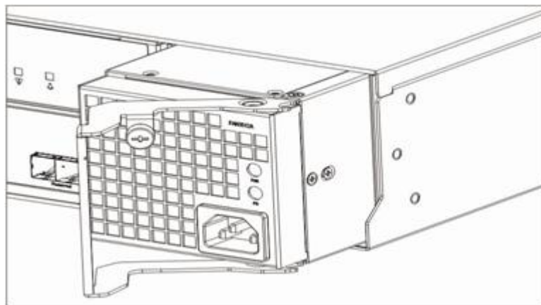
图6-18 安装/拆卸 DSU5625B 风扇模块+电池模块+电源模块示意图
