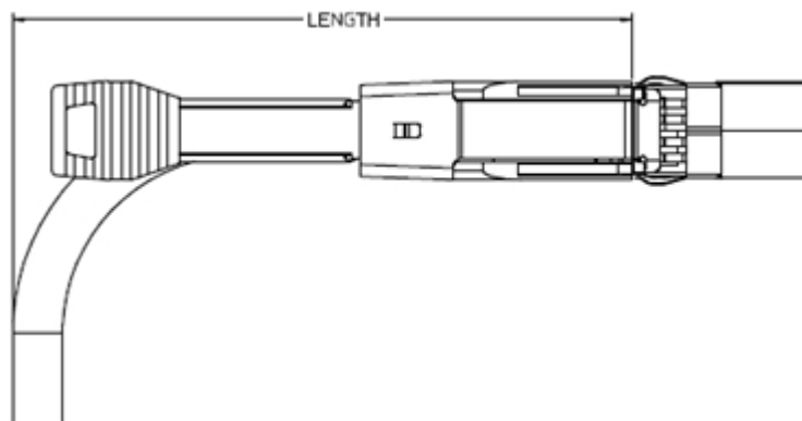
图4-37 铜缆弯曲半径示意图
