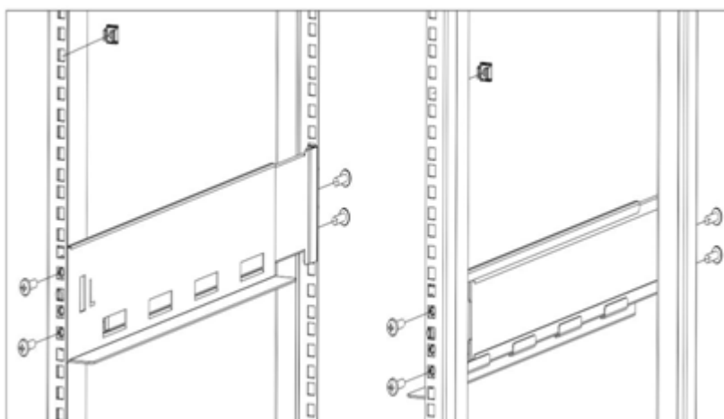
图4-11 安装浮动螺母示意图
