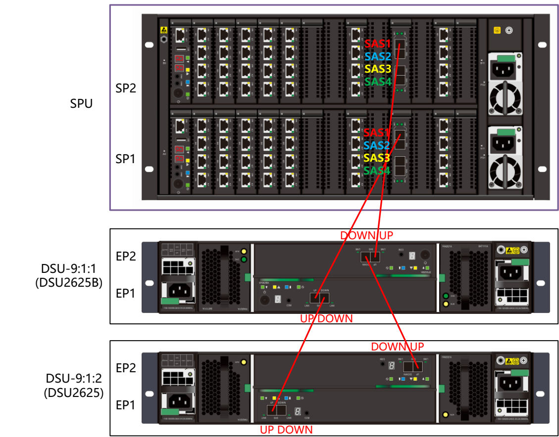
图4-39 SAS1 接口上 SAS 线缆安装示意图
