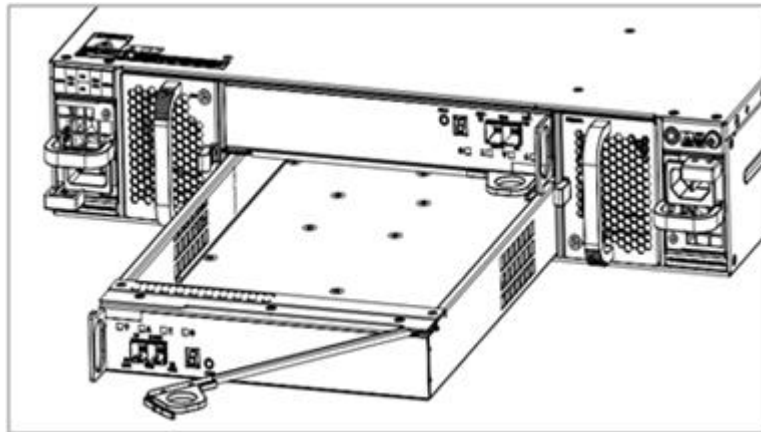
图6-6 安装/拆卸 DSU2625 EP 示意图
