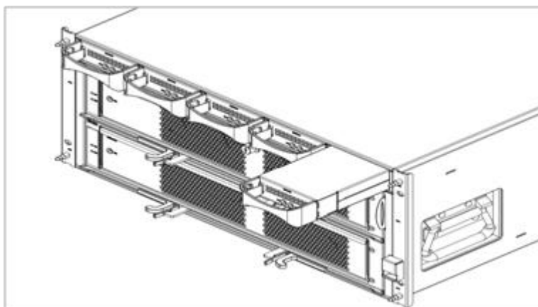
图4-14 安装 SPU 电池模块示意图
