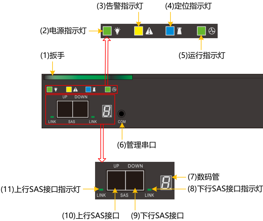
图3-13 DSU2625 的 EP 正视图
