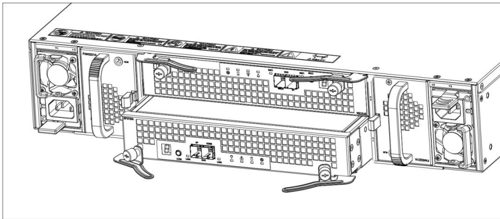
图6-8 安装/拆卸 DSU2725 EP 示意图
