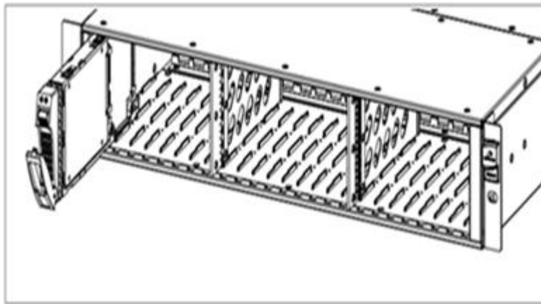
图6-25 安装 2.5 英寸磁盘模块 A 示意图（二）
