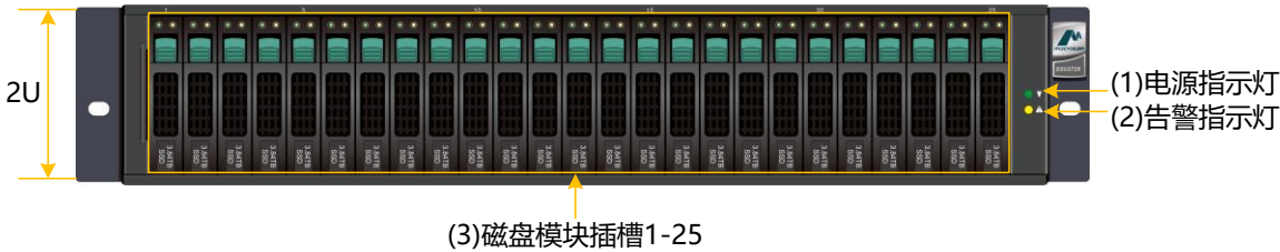
图3-28 DSU2725B/DSU2725 前正视图
