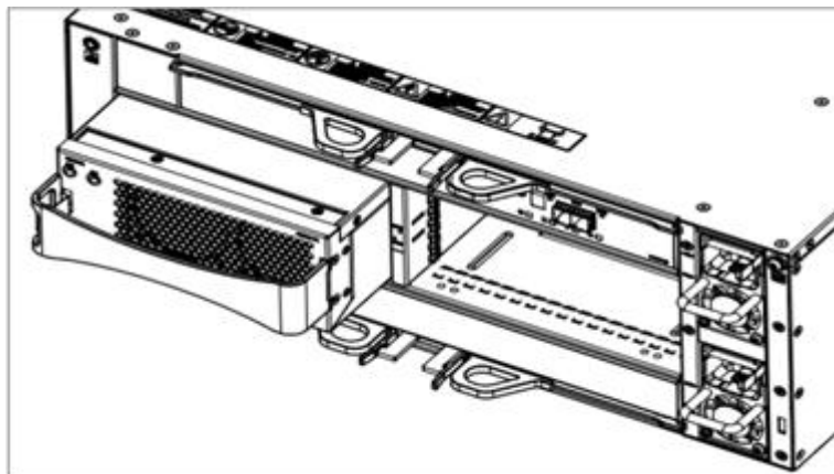
图6-14 安装/拆卸 DSU2624 风扇模块示意图
