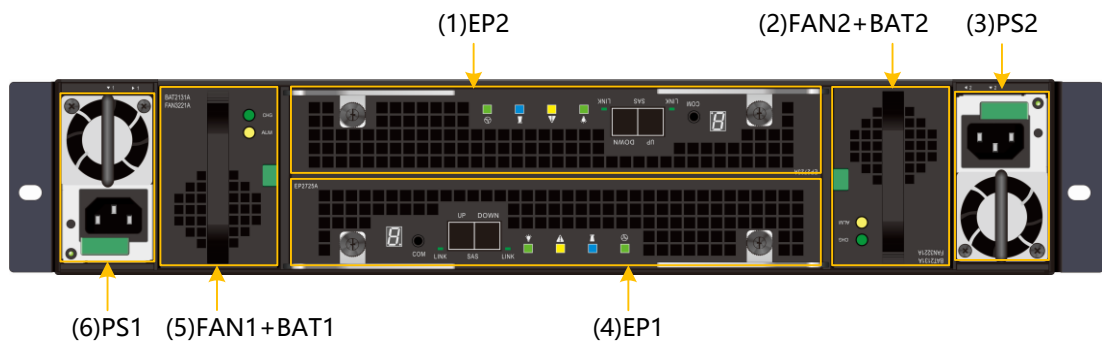
图3-29 DSU2725B 后正视图
