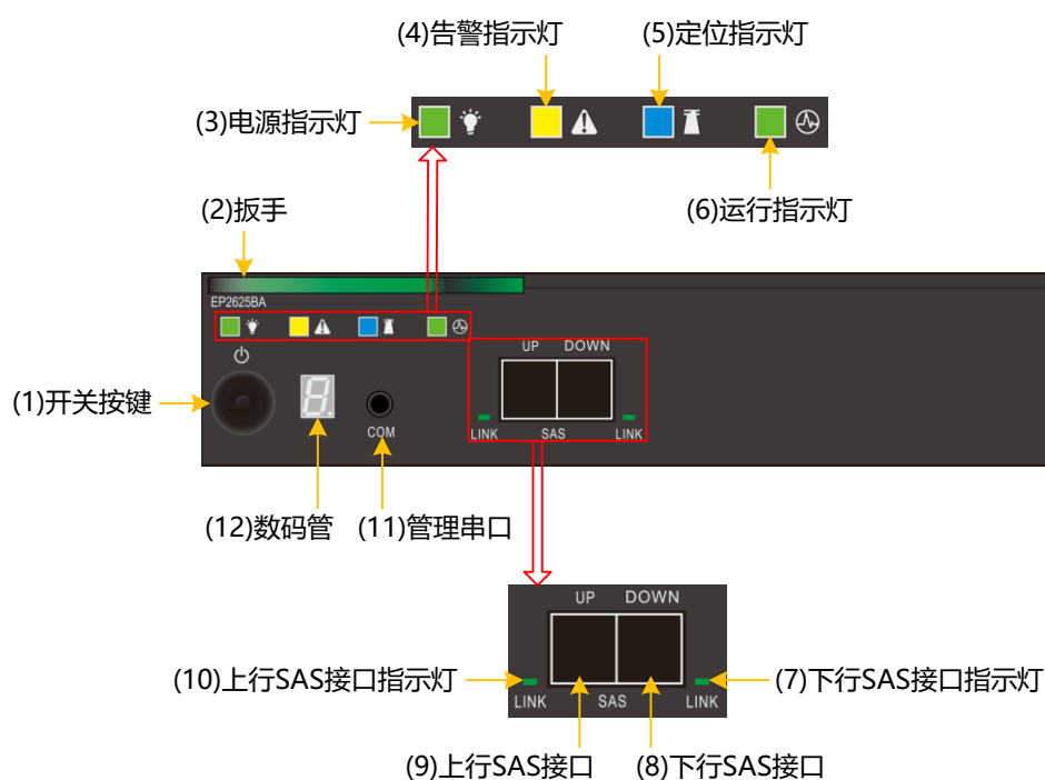
图3-12 DSU2625B 的 EP 正视图
