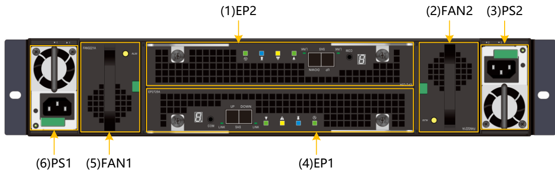
图3-30 DSU2725 后正视图
