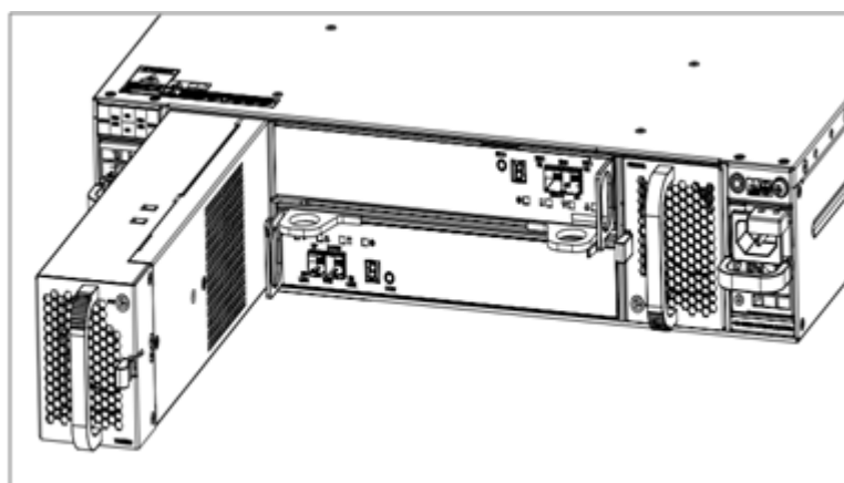
图4-18 安装 DSU2625B 风扇模块+电池模块示意图
