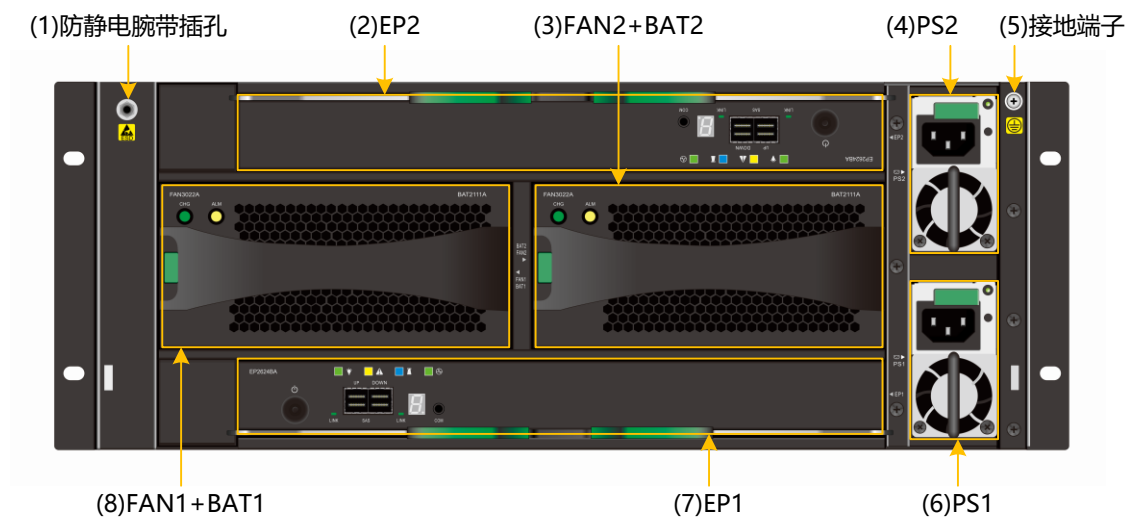
图3-20 DSU2624B 后正视图
