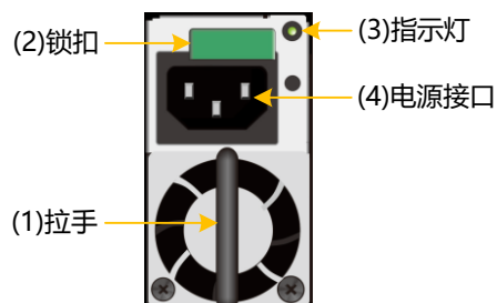
图3-36 DSU2725B/DSU2725 电源模块正视图
