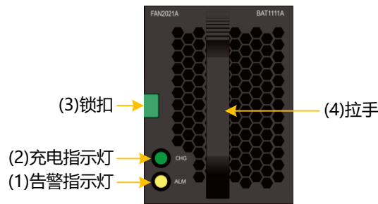
图3-14 DSU2625B 风扇模块+电池模块正视图
