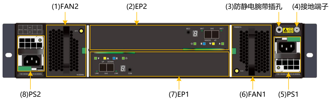
图3-11 DSU2625 后正视图
