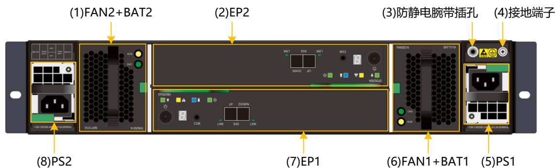
图3-10 DSU2625B 后正视图
