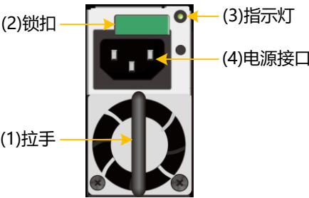
图3-8 SPU 电源模块正视图
