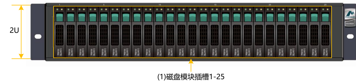
图3-39 DSU5625B/DSU5625 前正视图
