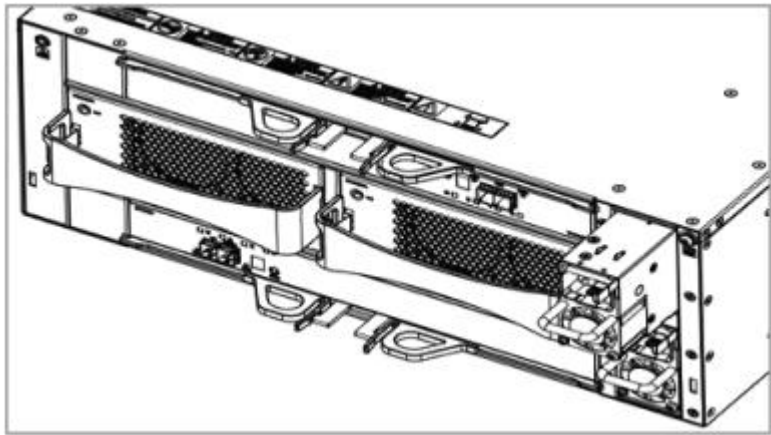
图6-21 安装/拆卸 DSU2624 电源模块示意图
