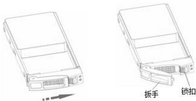
图6-28 安装 2.5 英寸磁盘模块 B 示意图（一）
