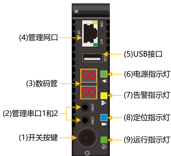
图3-5 SP 管理插卡正视图
