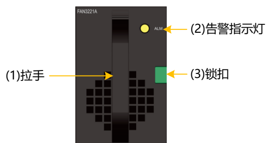
图3-35 DSU2725 后端风扇模块正视图
