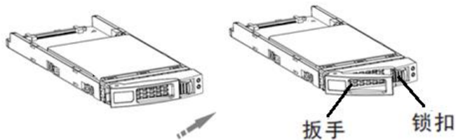
图6-24 安装 2.5 英寸磁盘模块 A 示意图（一）
