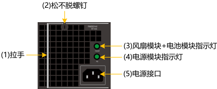
图3-43 DSU5625B 风扇模块+电池模块+电源模块正视图
