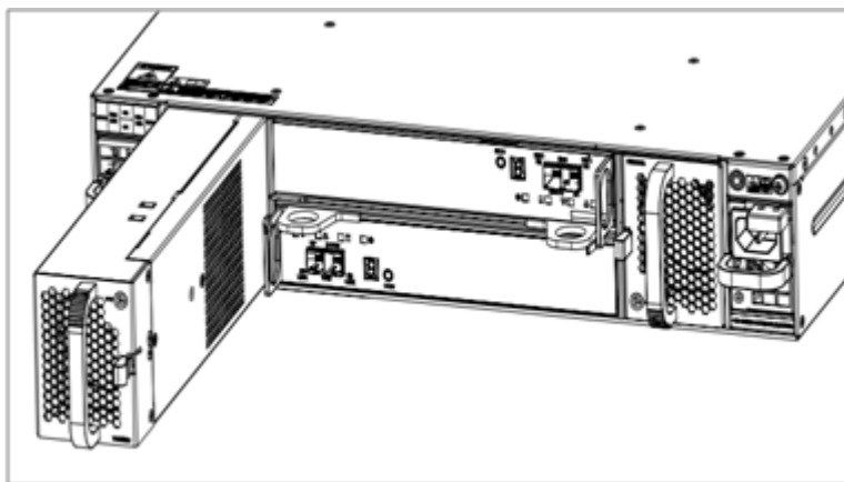
图6-10 安装/拆卸 DSU2625B 风扇模块+电池模块示意图
