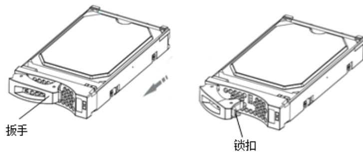
图6-32 安装 3.5 英寸磁盘模块示意图（一）
