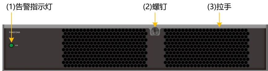
图3-6 SPU 风扇模块正视图
