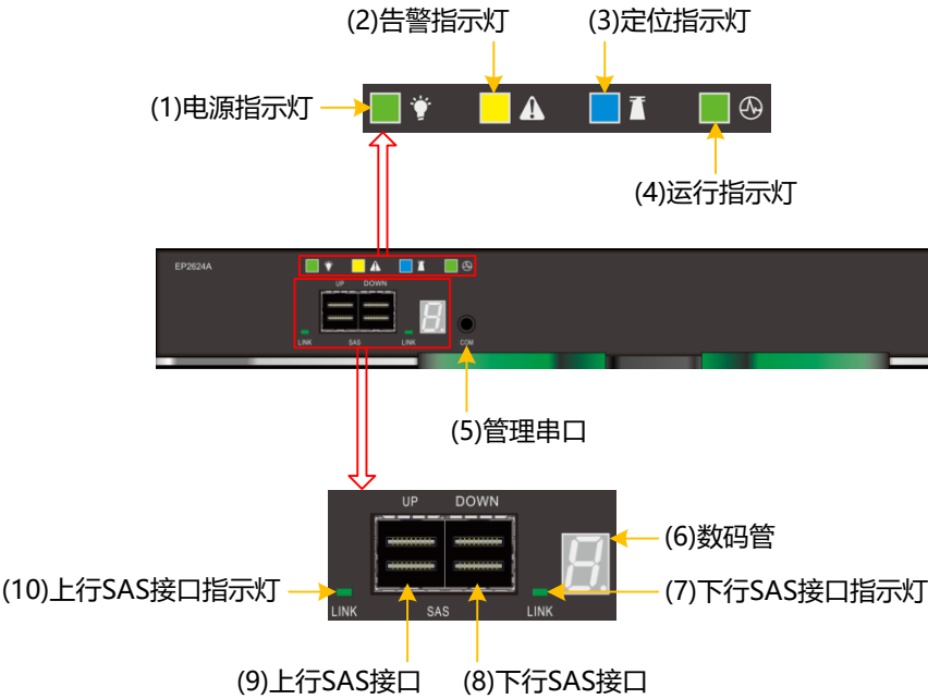
图3-23 DSU2624 的 EP 正视图
