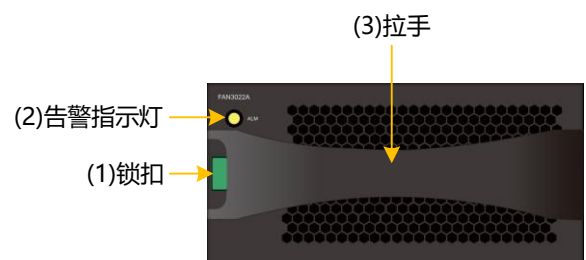
图3-25 DSU2624 风扇模块正视图
