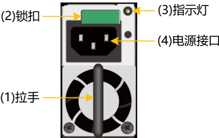
图3-26 DSU2624B/DSU2624 电源模块正视图
