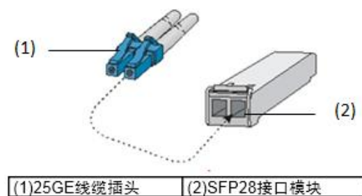
图4-45 25GE 线缆和接口示意图
