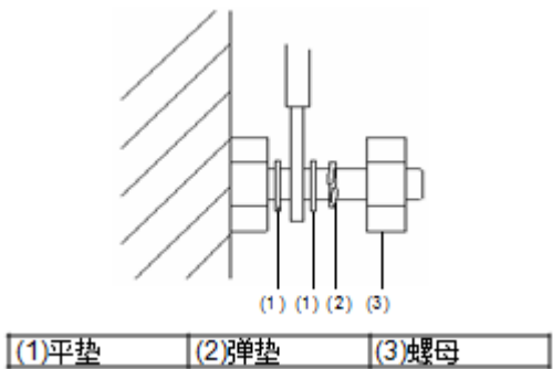
图4-22 固定线缆端子示意图
