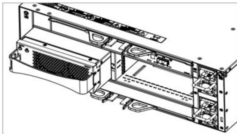
图6-11 安装/拆卸 DSU2624B 风扇模块+电池模块示意图
