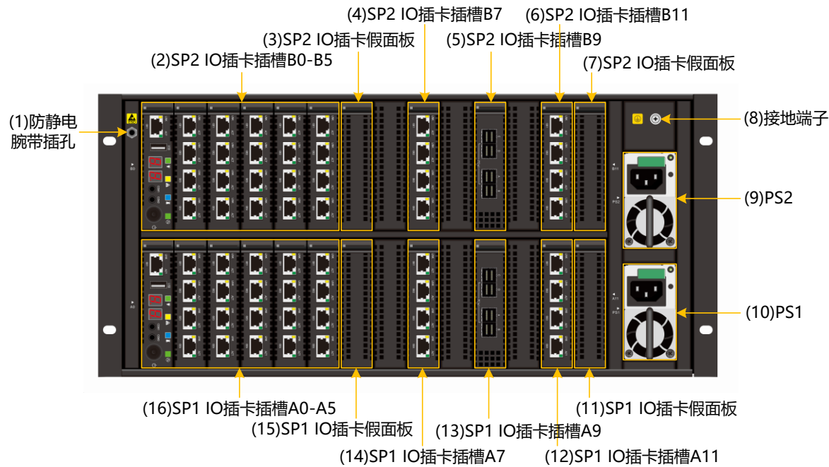
图3-3 SPU 后正视图
