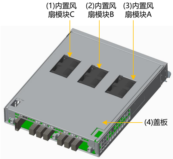
图3-33 DSU2725B/DSU2725 内置风扇模块安装位置示意图
