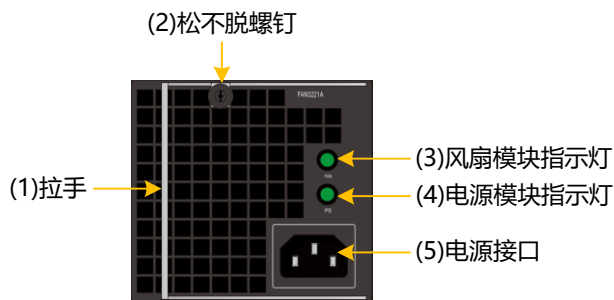
图3-44 DSU5625 风扇模块+电源模块正视图
