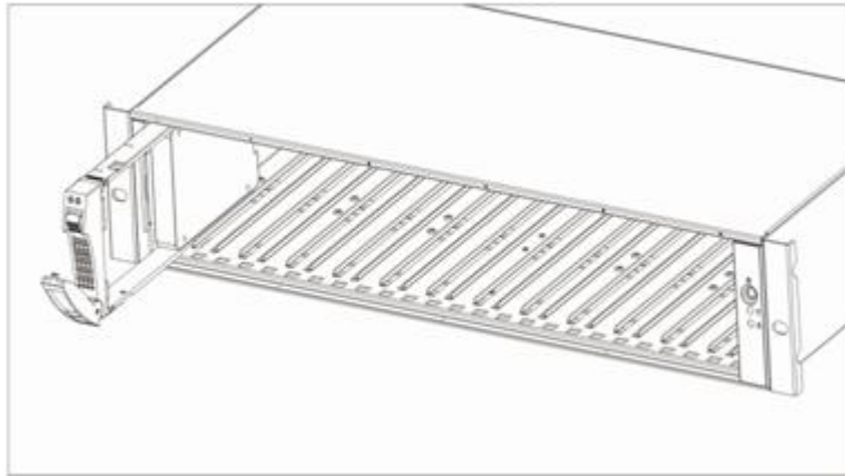
图6-37 安装 NVMe 磁盘模块示意图（二）
