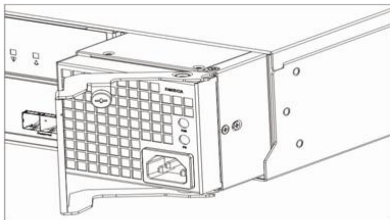
图6-20 安装/拆卸 DSU5625 风扇模块+电源模块示意图
