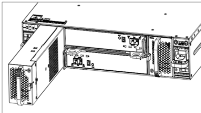
图6-13 安装/拆卸 DSU2625 风扇模块示意图
