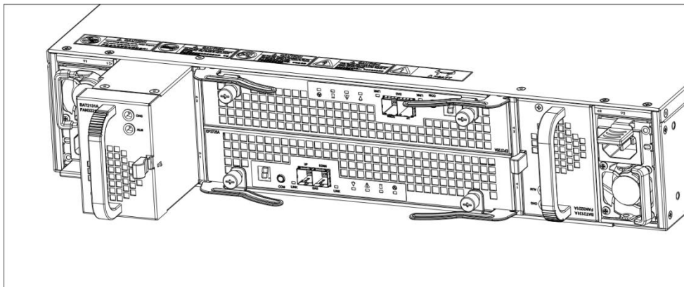
图4-20 安装 DSU2725B 风扇模块+电池模块示意图
