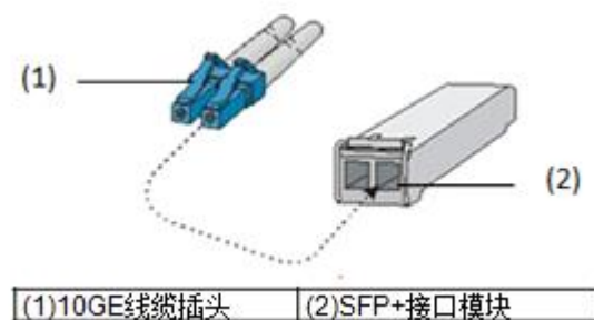
图4-44 10GE 线缆和接口示意图
