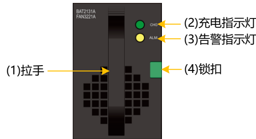
图3-32 DSU2725B 风扇模块+电池模块正视图
