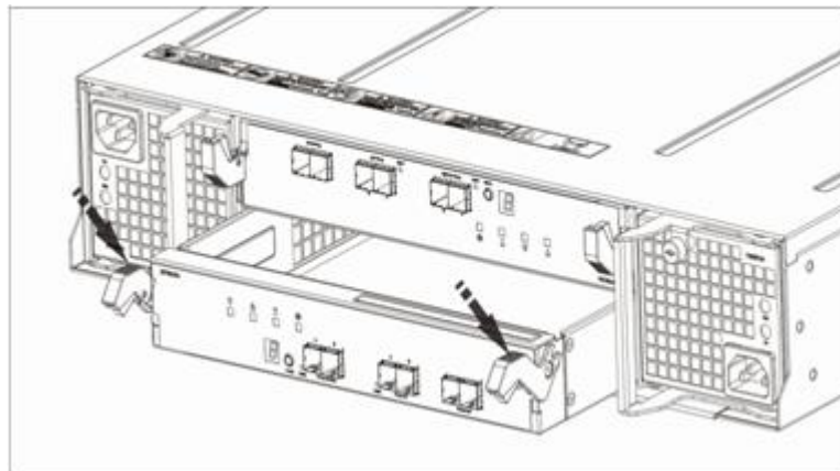
图6-9 安装/拆卸 DSU5625 EP 示意图
