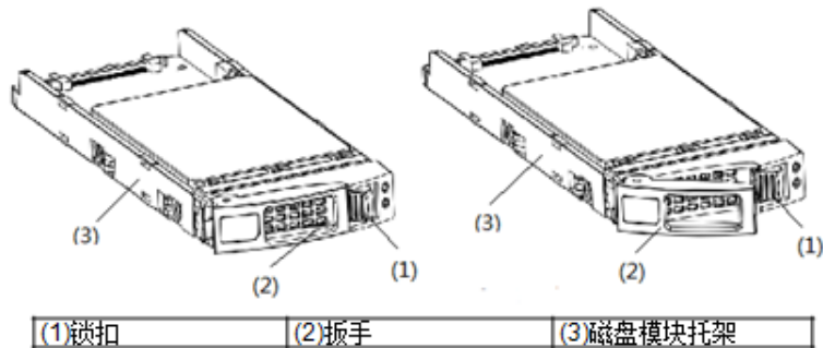
图6-22 2.5 英寸磁盘模块 A 示意图
