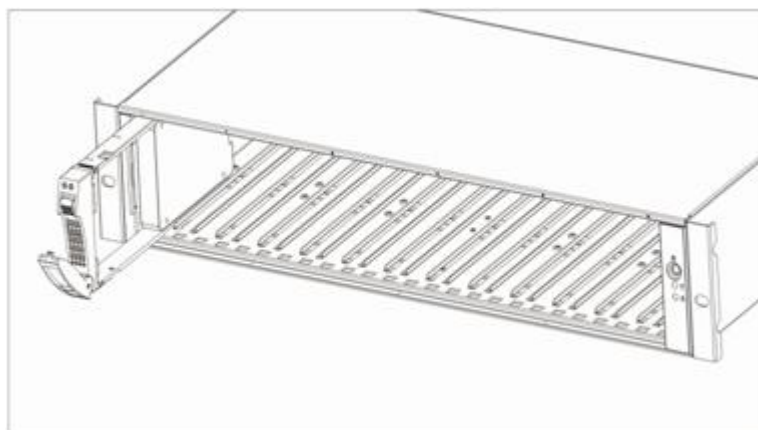
图6-29 安装 2.5 英寸磁盘模块 B 示意图（二）
