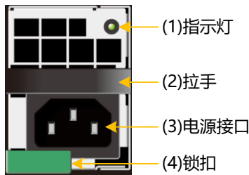
图3-16 DSU2625B/DSU2625 电源模块正视图
