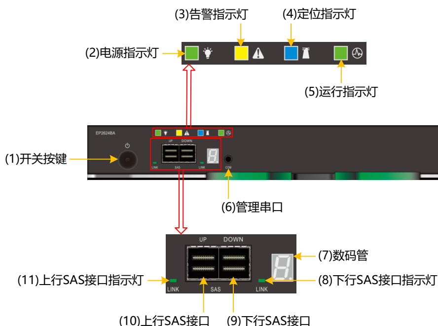
图3-22 DSU2624B 的 EP 正视图
