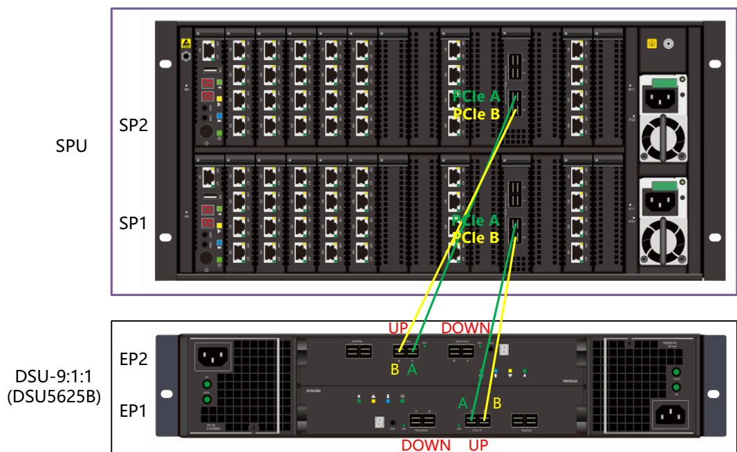
图4-41 PCIe 扩展线缆安装示意图
