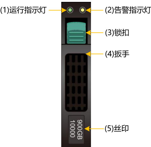
图3-38 2.5 英寸磁盘模块前面板
