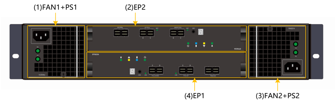
图3-41 DSU5625 后正视图
