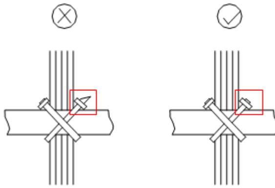
图4-24 线缆捆扎示意图（二）
