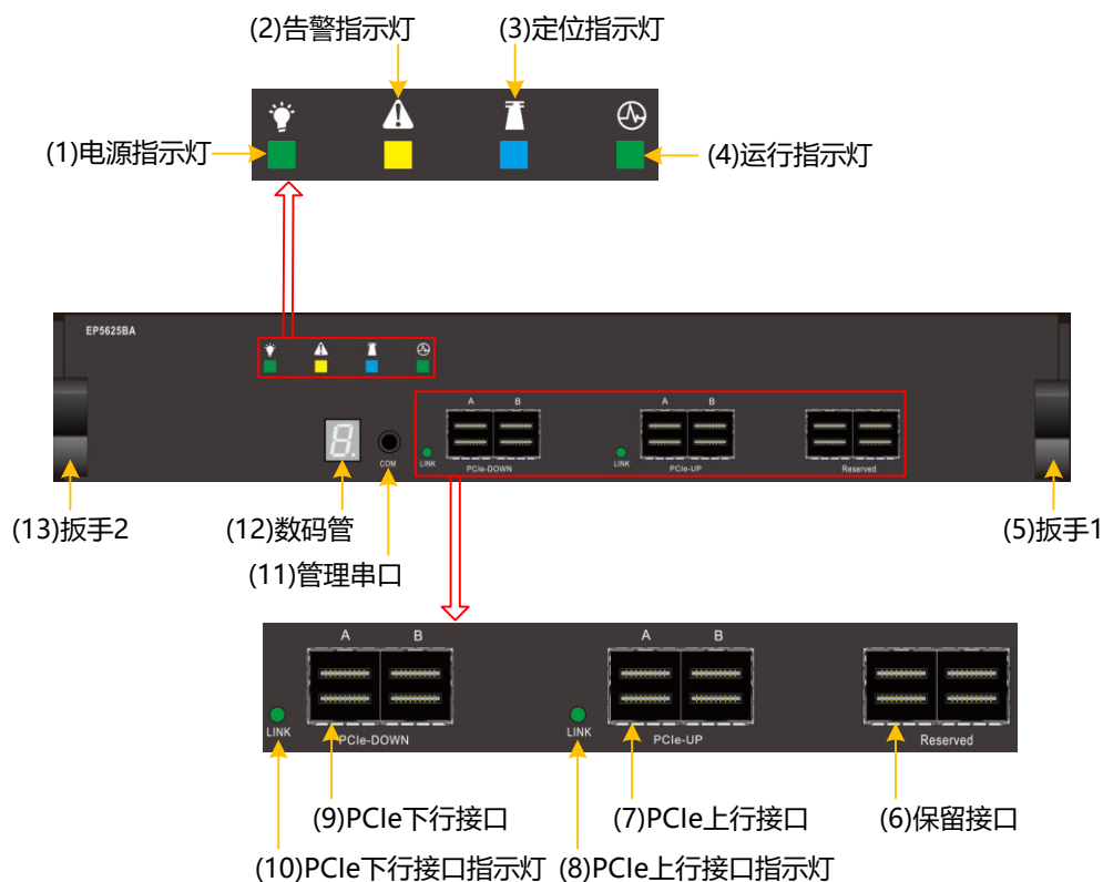
图3-42 DSU5625B/DSU5625 的 EP 正视图
