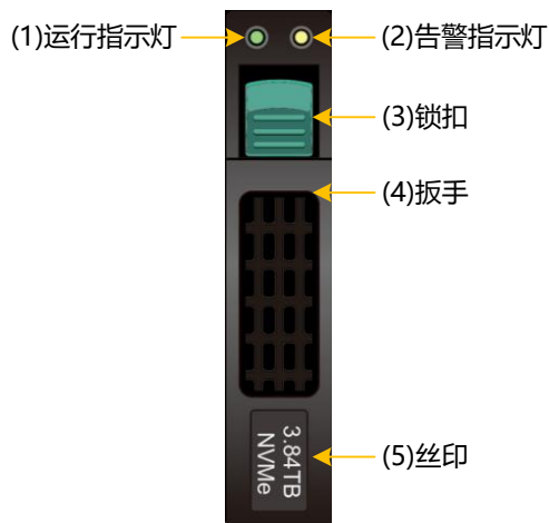
图3-45 NVMe 磁盘模块前面板
