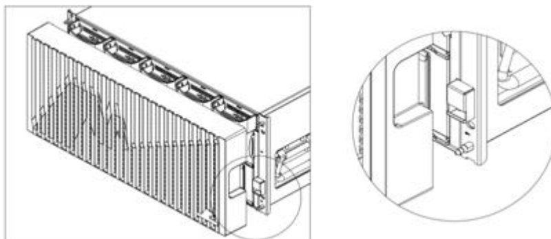
图6-1 安装/拆卸 SPU 面板示意图
