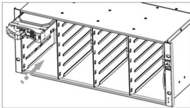
图6-33 安装 3.5 英寸磁盘模块示意图（二）
