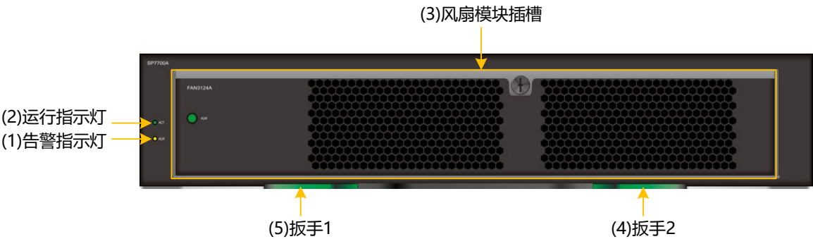
图3-4 SP 正视图
