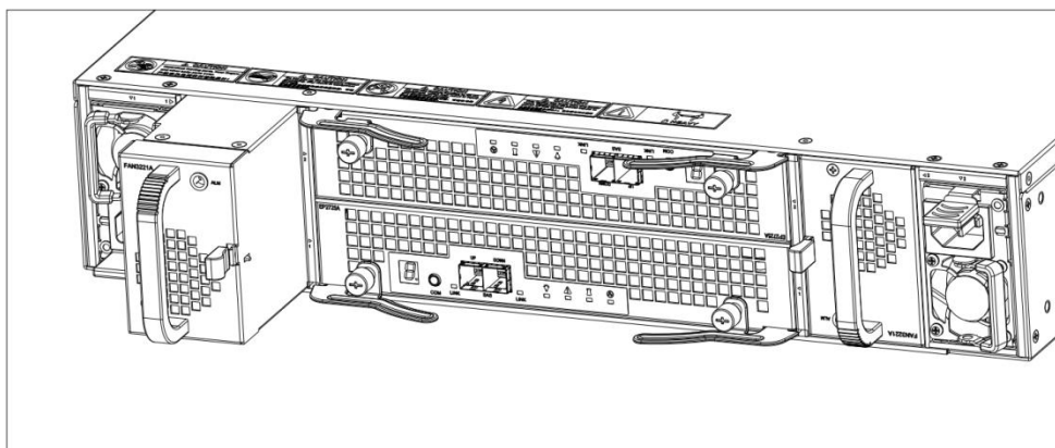
图6-17 安装/拆卸 DSU2725 后端风扇模块示意图
