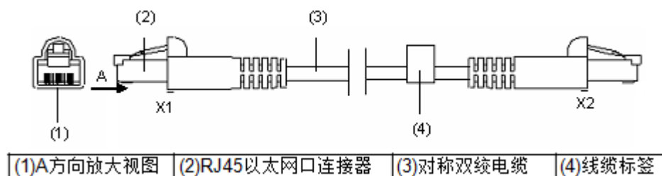
图4-43 GE 线缆示意图
