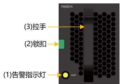
图3-15 DSU2625 风扇模块正视图
