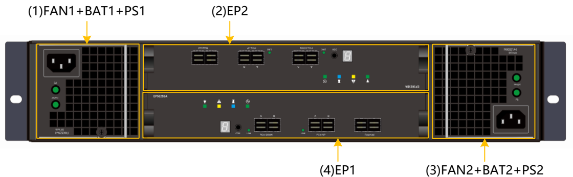
图3-40 DSU5625B 后正视图
