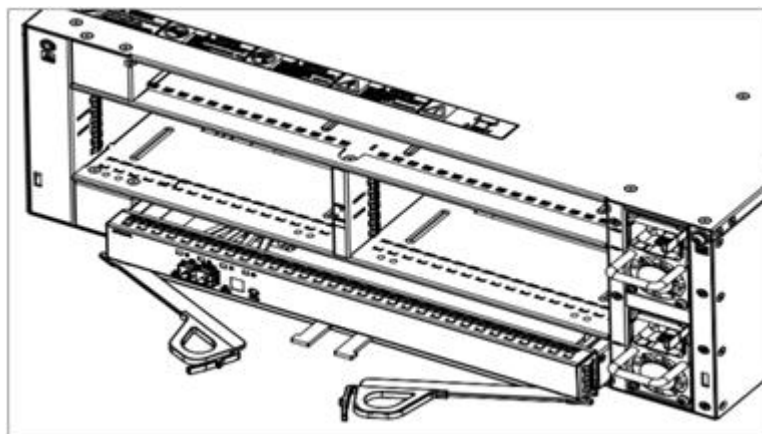
图6-7 安装/拆卸 DSU2624 EP 示意图
