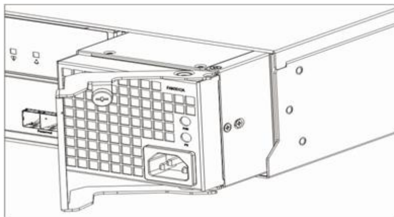
图4-21 安装 DSU5625B 风扇模块+电池模块+电源模块示意图
