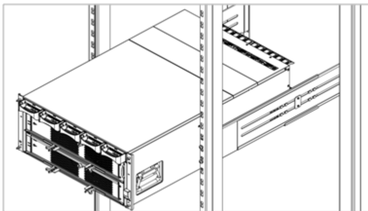
图4-13 安装 SPU 示意图
