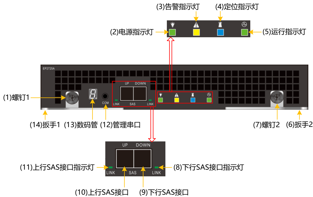
图3-31 DSU2725B/DSU2725 的 EP 正视图
