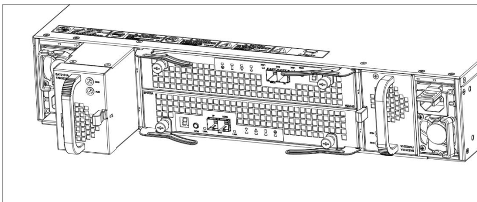
图6-12 安装/拆卸 DSU2725B 风扇模块+电池模块示意图
