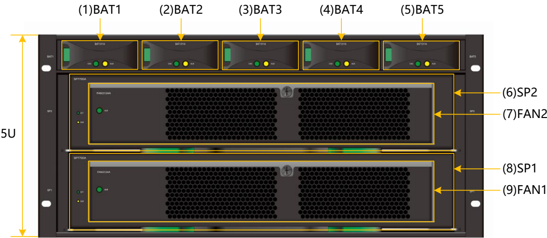
图3-2 SPU 前正视图（不带面板）
